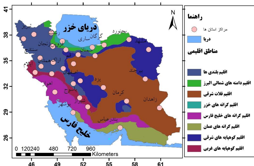
شکل ۱- پراکندگی مناطق اقلیمی کشور (Masoudian, 2007)
