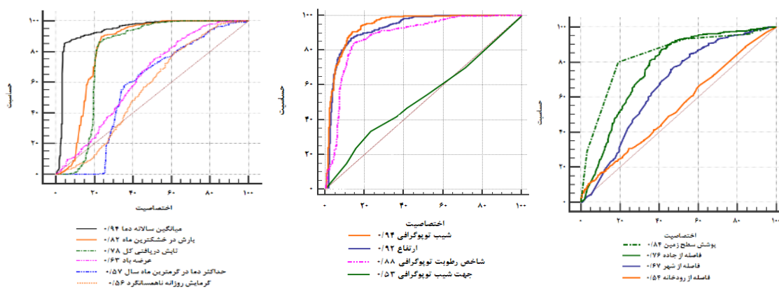
شکل ۵- نمودارهای راک عوامل مؤثر بر احتمال حساسیت آتش‌سوزی جنگل‌ها و مراتع در روش شبکه عصبی
