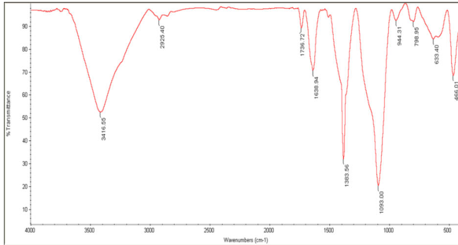
شکل ۲- طیف FT- IR نانوکامپوزیت \text{Fe}_3\text{O}_4/\text{SiO}_2 اصلاح شده
