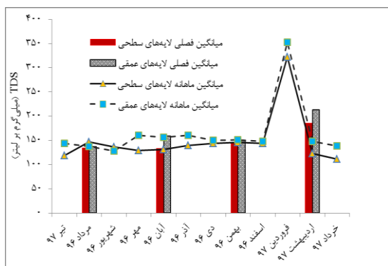
شکل ۴- تغییرات میانگین ماهانه و فصلی کدورت و مواد جامد محلول در لایه‌های مختلف دریاچه سد گاران، ۱۳۹۶-۱۳۹۷.
